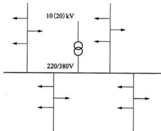
图 D.0.2 树干型
