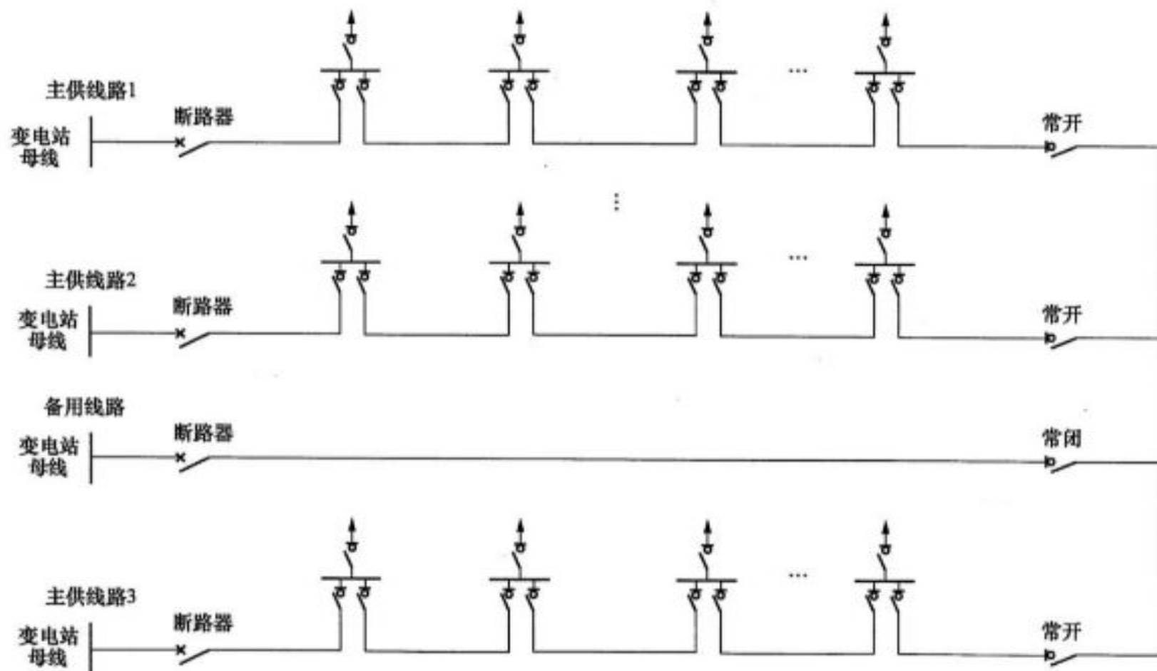
图 C.0.2-3 N 供一备 ( 2 \leq N \leq 3 )
