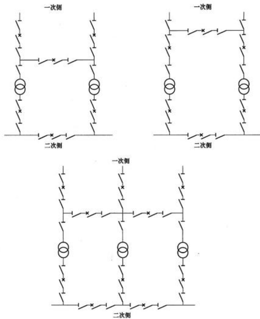
图 B.0.3 桥式（内桥、外桥、扩大内桥）
