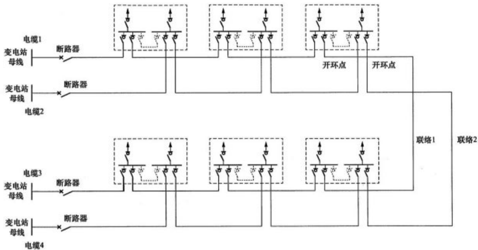
图 C.0.2-2 双环式
