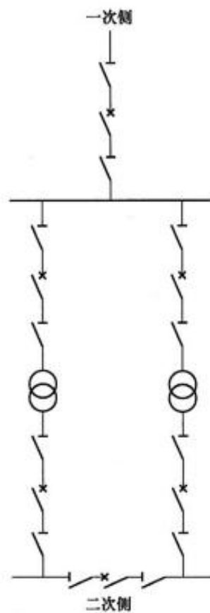
图 B.0.1 单母线
