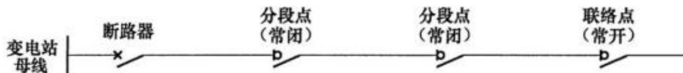
图 C.0.1-2 多分段单联络
