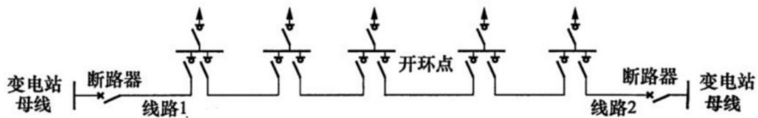
图 C.0.2-1 单环式
