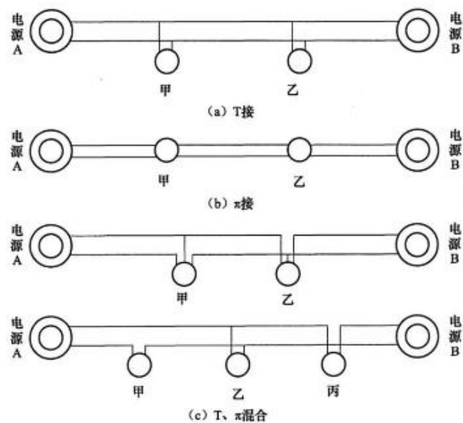
图 A.0.3-2 双链
