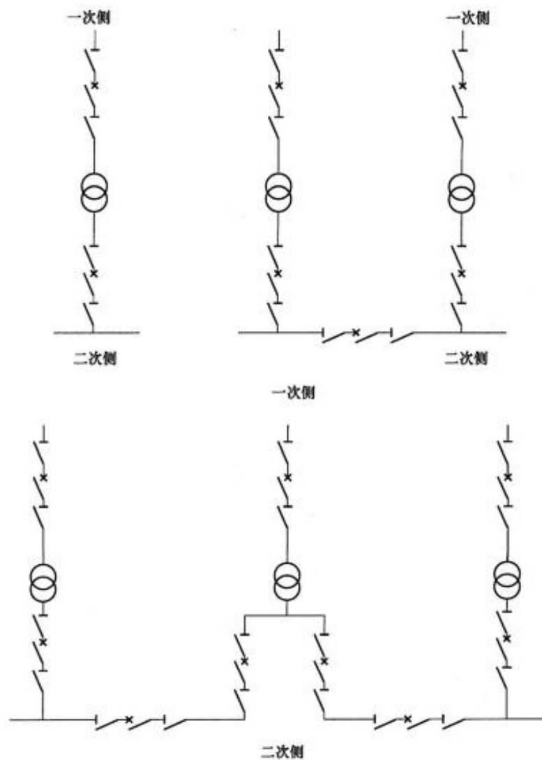
图 B.0.4 线变组
