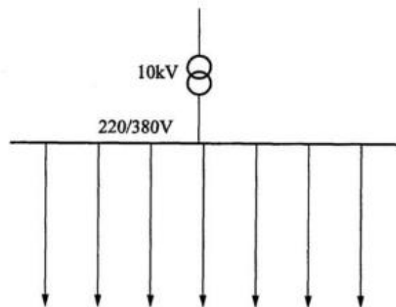
图 D.0.1 放射型
