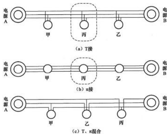
图 A.0.3-3 三链
