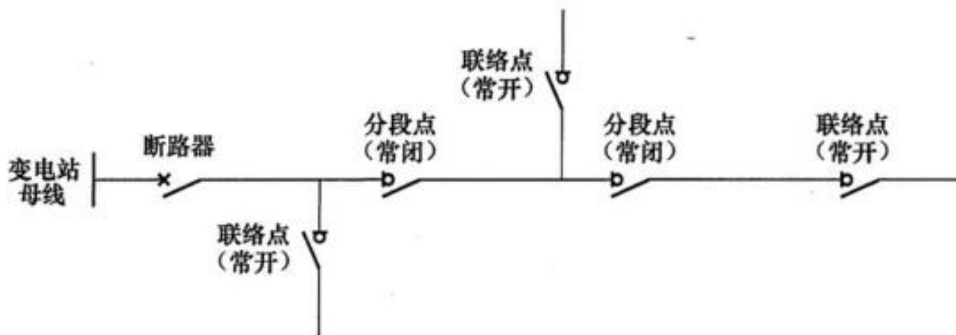
图 C.0.1-3 多分段适度联络
