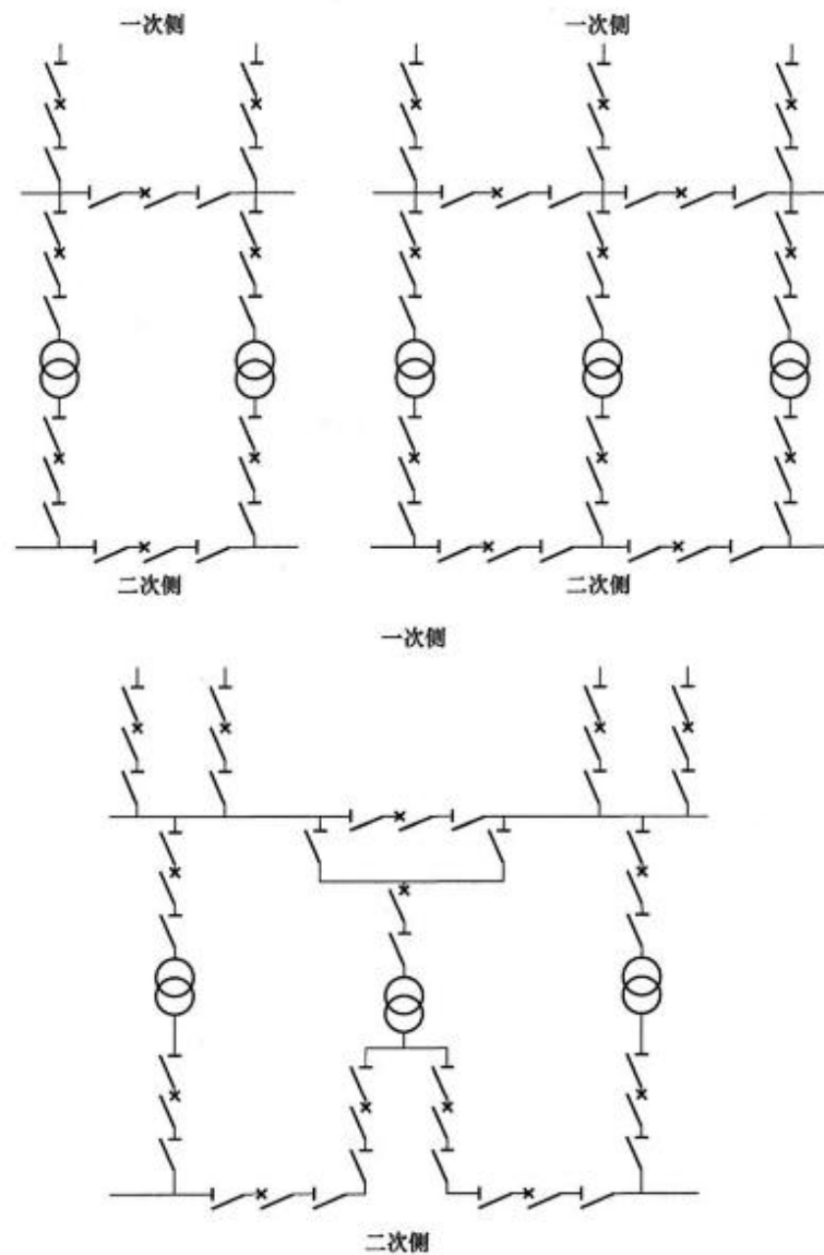
图 B.0.2 单母线分段
