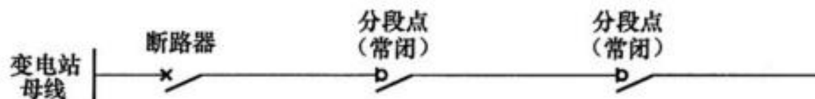
图 C.0.1-1 多分段单辐射
